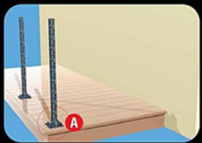
1. ติดตั้งเสาเหล็กชุบกันสนิม พร้อมเหล็กรับราระเบียงตามระยะของขนาดราระเบียงไม้เนื้อมาตรฐาน (1.0, 1.5, 2.0 เมตร)
